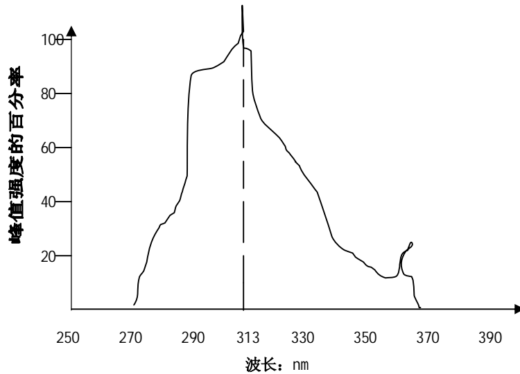
图3 UV-B 荧光紫外灯的相对分光光谱辐照度
